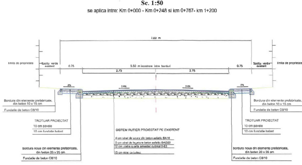
PROFIL TRANSVERSAL TIP NR.1
