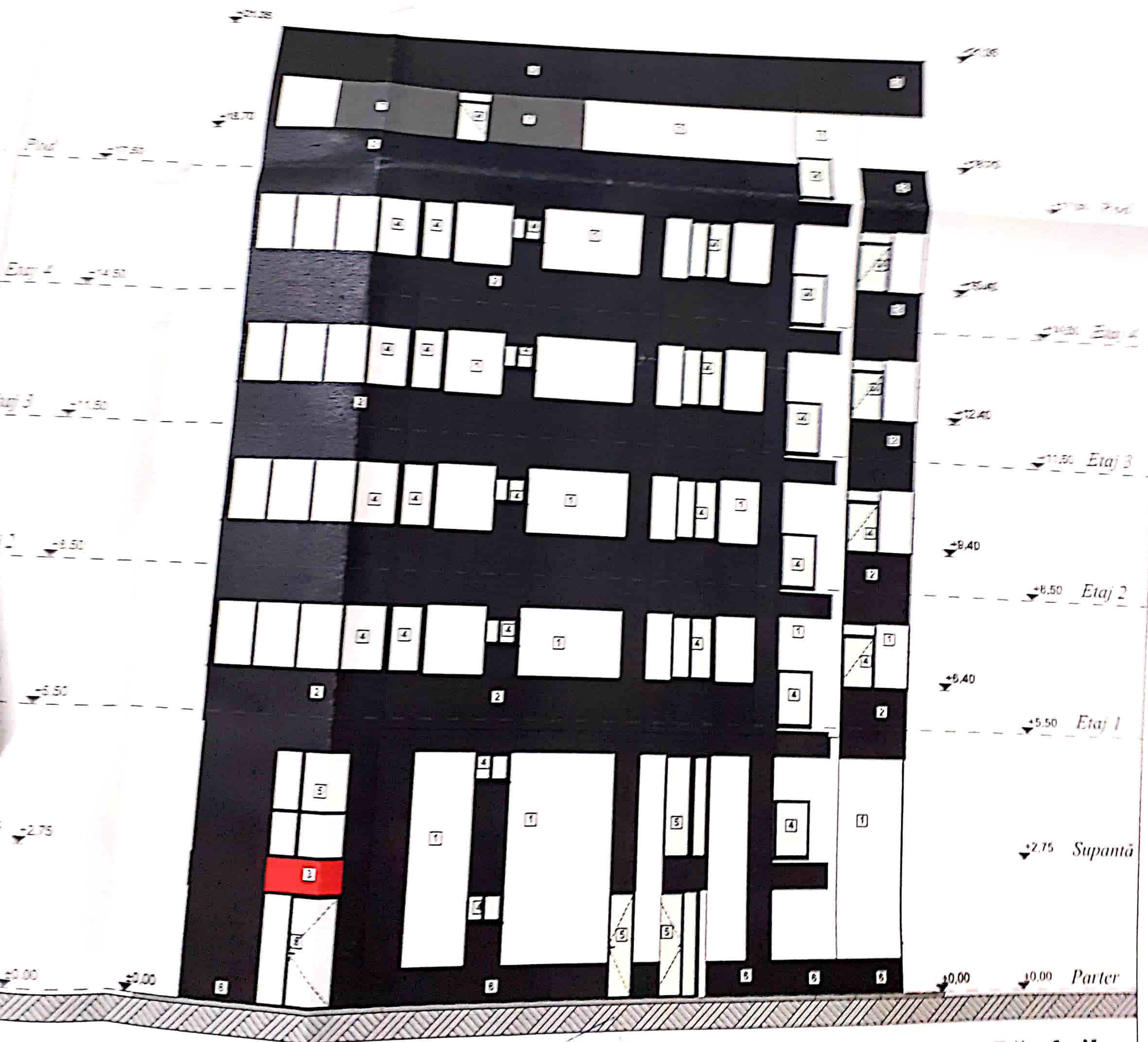
Fațadă lateral dreapta -(est) str. Bătrânilor 1:100
