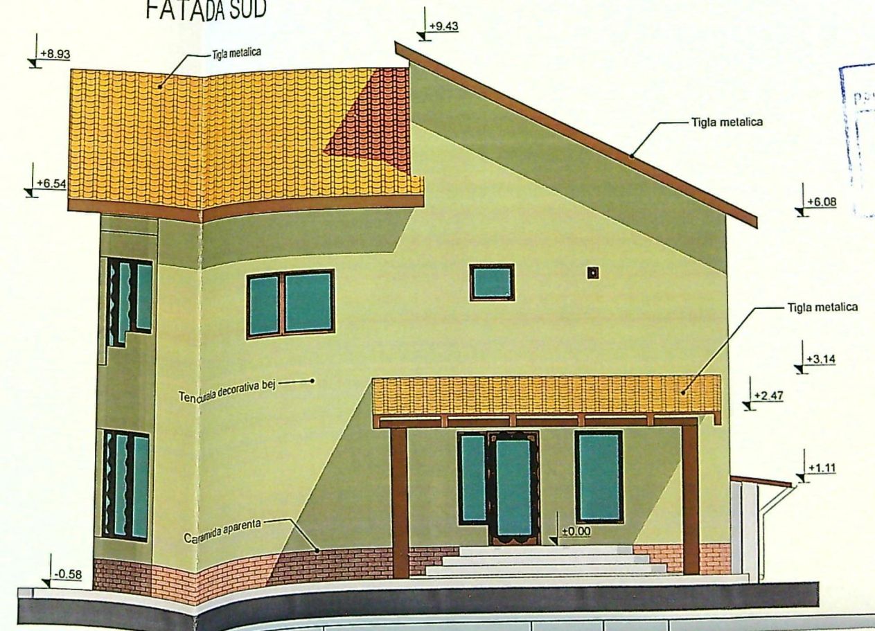
FATADA EST
