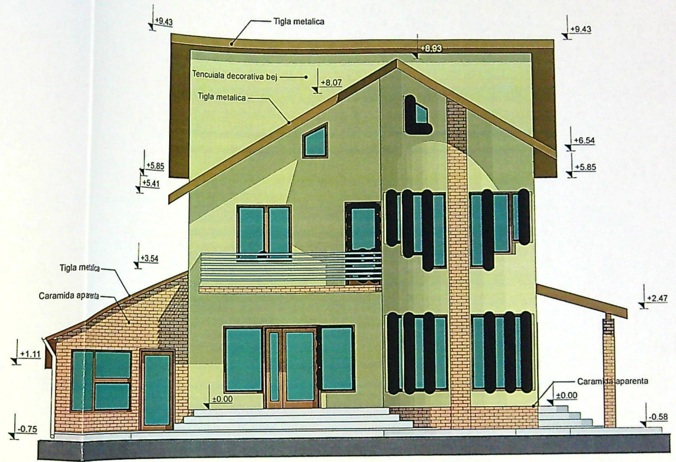
FATADA SUD
