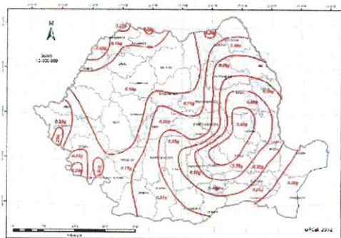
Figura A1 România - Zonarea valorilor de vârf ale accelerației terenului pentru proiectare cu IMR = 225 ani și 20% probabilitate de depășire în 50 de ani.
