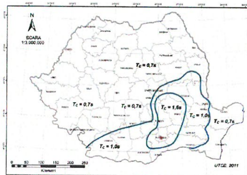
Figura A2 Zonarea teritoriului României în termeni de perioadă de control (colt), T_c a spectrului de răspuns
