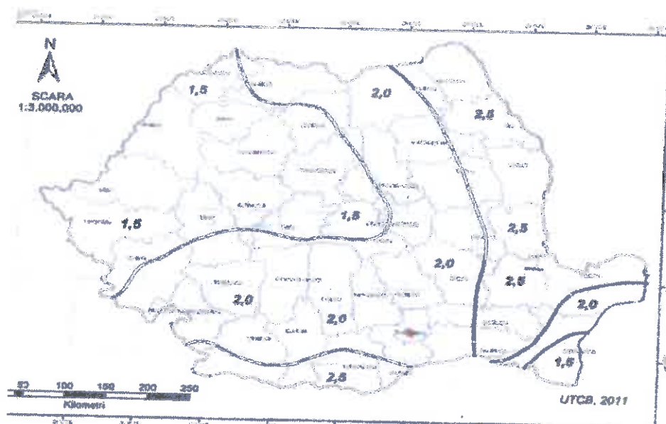
1. Zonarea valorilor caracteristice ale încărcării din zăpada pe sol s_s , \text{kN/m}^2 , pentru altitudini A \approx 1000 \text{ m} NOTA: Pentru altitudini A > 1000 \text{ m} valorile s_s se determina cu relatiile (3.1) si (3.2)
