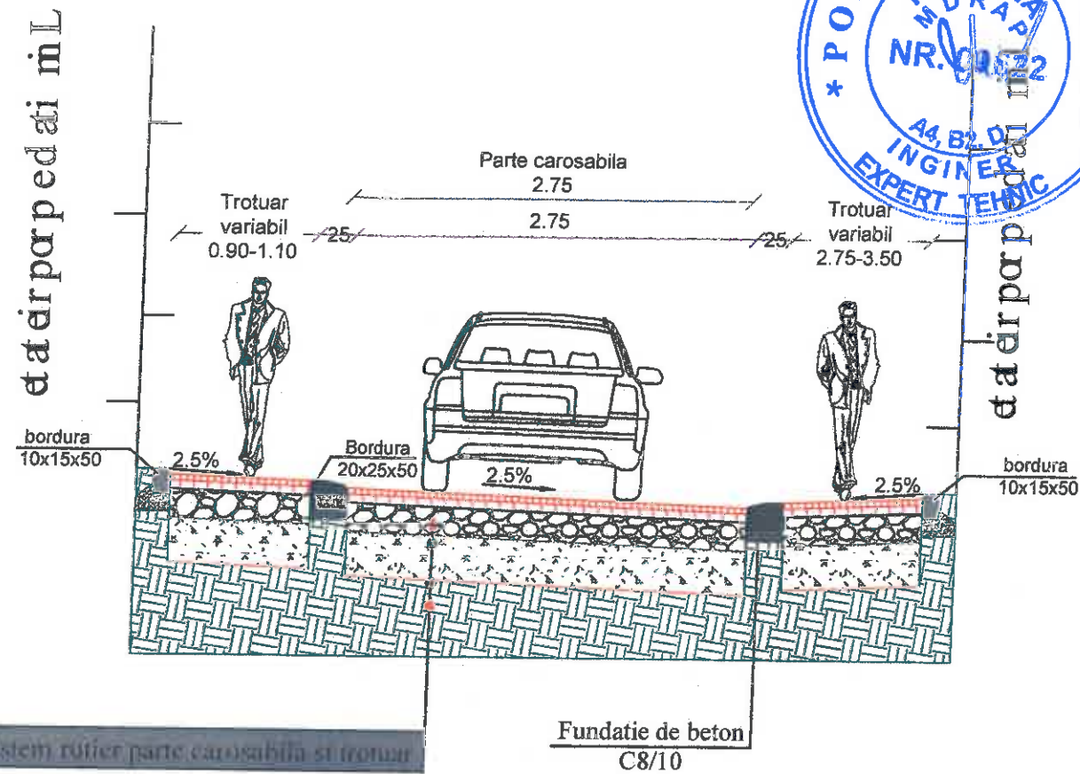
Profil transversal TIP 3
